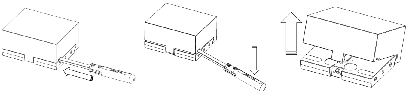
Abb. 17 Darstellung zur fachgerechten Abnahme der Aufsatzbacke von der Grundbacke
