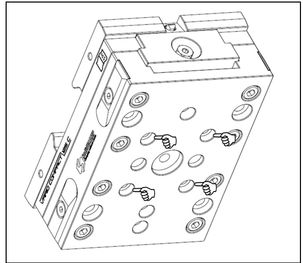
Abb. 21 Aufnahmen für Nullpunktsystem mit Maß 52
