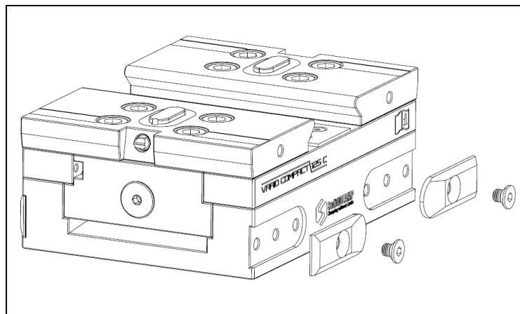
Abb. 19 Seitliche Designkappen entfernen
