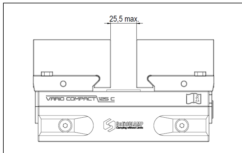
Abb. 6 Maximaler Hub bei aufgesetzten Aufsatzbacken Vario Compact 125 C
