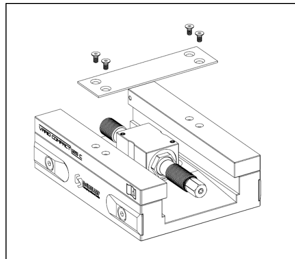
Abb. 13 Schutzblech entfernen
