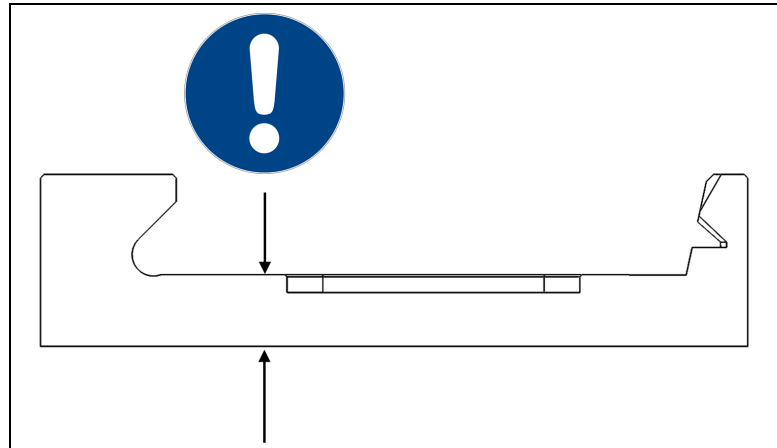
Abb. 28 Hinweis auf eine nicht zu gering werdende Bodenstärke der Aufsatzbacke
