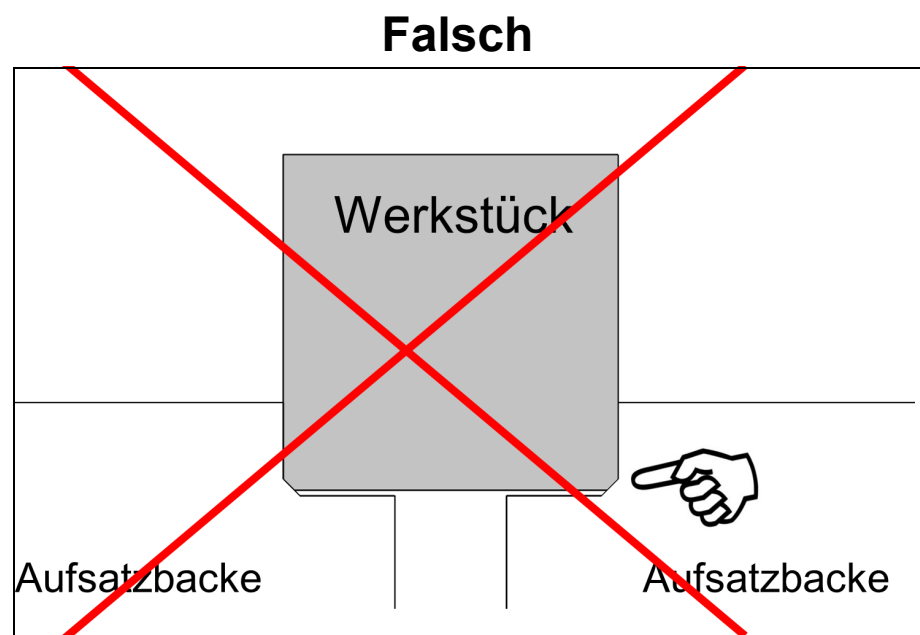
Abb. 24 Darstellung einer falschen Spannung. Der Kantenbruch der Kontur in der Aufsatzbacke ist größer als der Kantenbruch des zu spannenden Werkstücks
