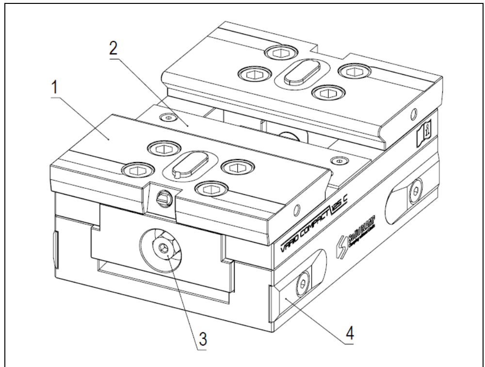
Abb. 4 Beschreibung Vario Compact 125 C
