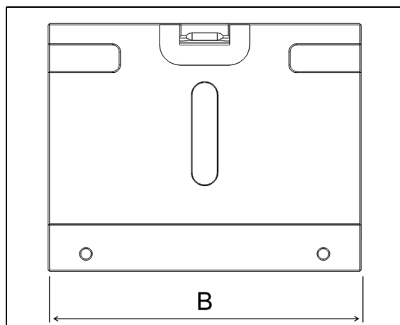
Abb. 3 Aufsatzbacke mit Darstellung der Backenbreite
