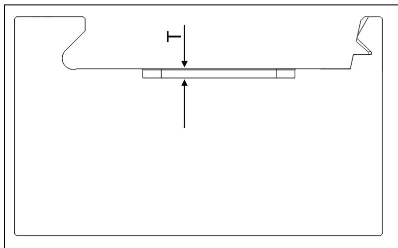
Abb. 2 Schnitt durch Aufsatzbacke zur Darstellung der Passfedernut-Tiefe
