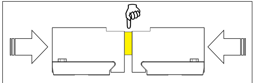
Abb. 23 Eingespanntes paralleles Distanzstück (gelb) direkt unterhalb der ausgefrästen Kontur
