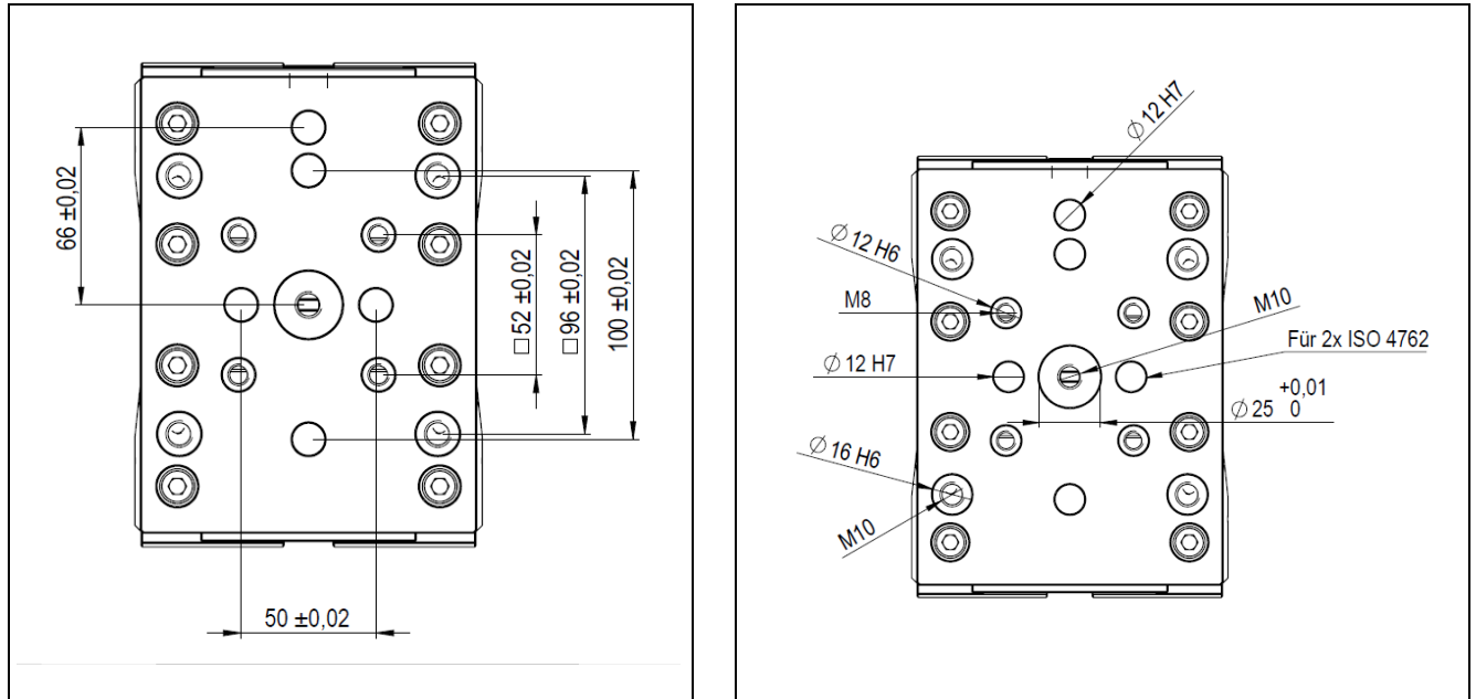
Abb. 7 Anschlusschnittstellen Unterseite Vario Compact 125 C
