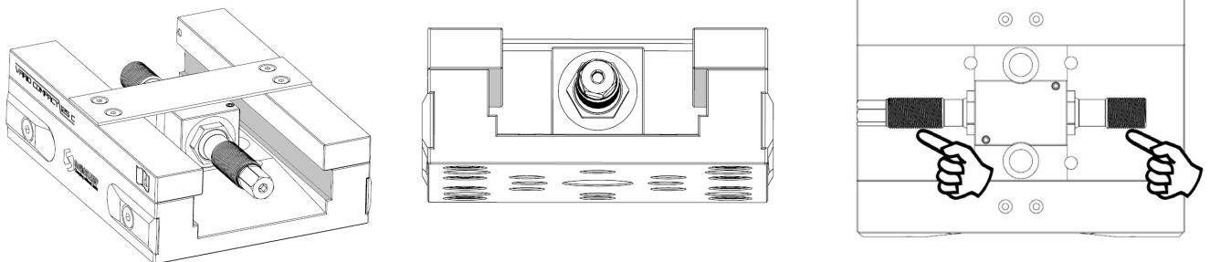
Abb. 30 Darstellung der zu schmierenden Flächen am Vario Compact 125 C. Die in der Darstellung grau oder mit einem Finger markierten Flächen sind zu schmieren
