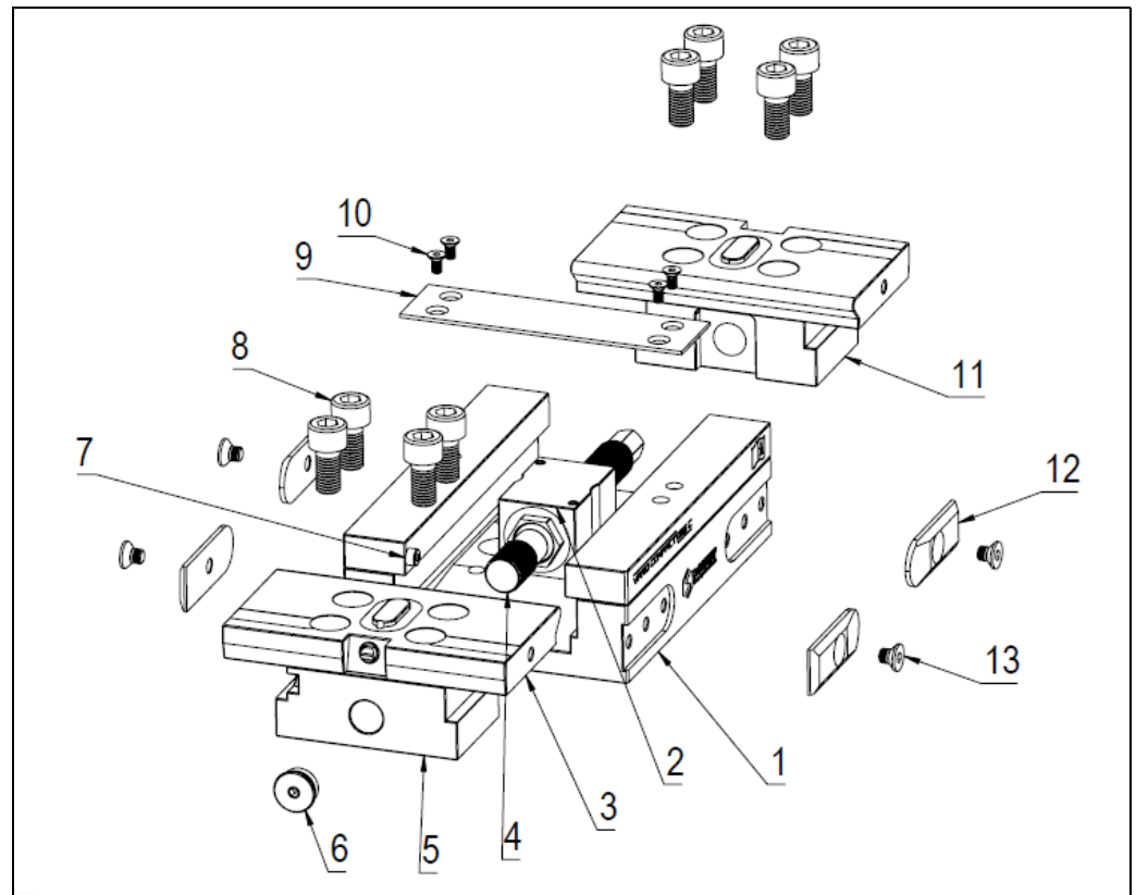
Abb. 32 Explosionsdarstellung Vario Compact 125 C
