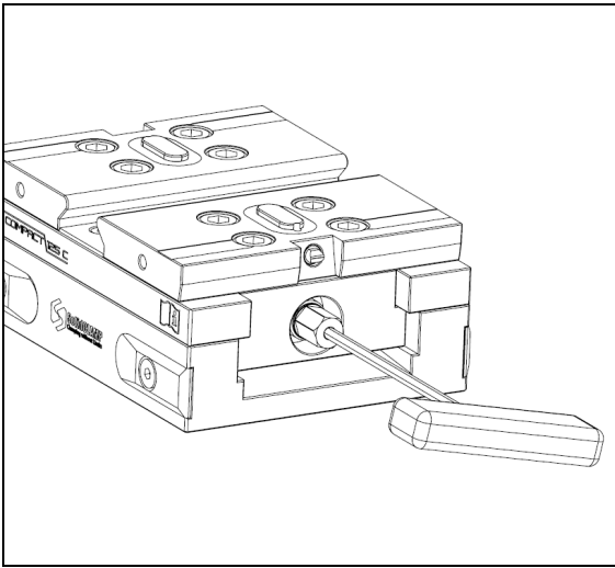
Abb. 10 Schieber nach Innen fahren
