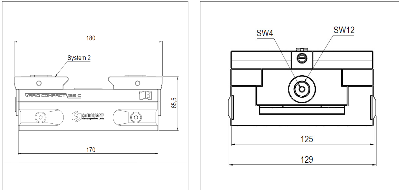
Abb. 5 Allgemeine Außenmaße Vario Compact 125 C
