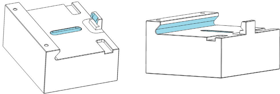
Abb. 31 Darstellung der zu schmierenden Flächen der Aufsatzbacke. Die in der Darstellung türkis markierten Flächen sind zu schmieren
