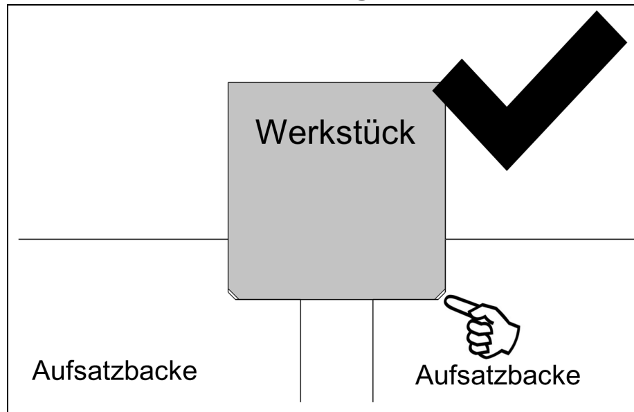
Abb. 25 Darstellung einer richtigen Spannung. Der Kantenbruch der Kontur in der Aufsatzbacke ist kleiner als der Kantenbruch des zu spannenden Werkstücks
