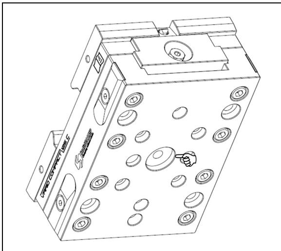
Abb. 22 Aufnahme für Nullpunktsystem mit mittiger Einzelspannaufnahme
