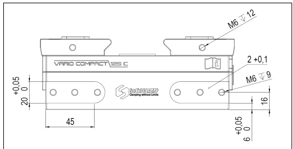
Abb. 8 Anschlusschnittstelle Seite Vario Compact 125 C
