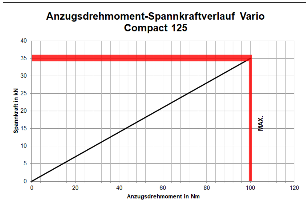
Abb. 1 Spannkraftverlauf Vario Compact 125 C
