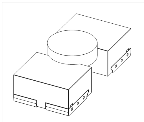
Darstellung eines ungünstigen Falls. Es ist ein großer Spalt zwischen den Aufsatzbacken vorhanden.
