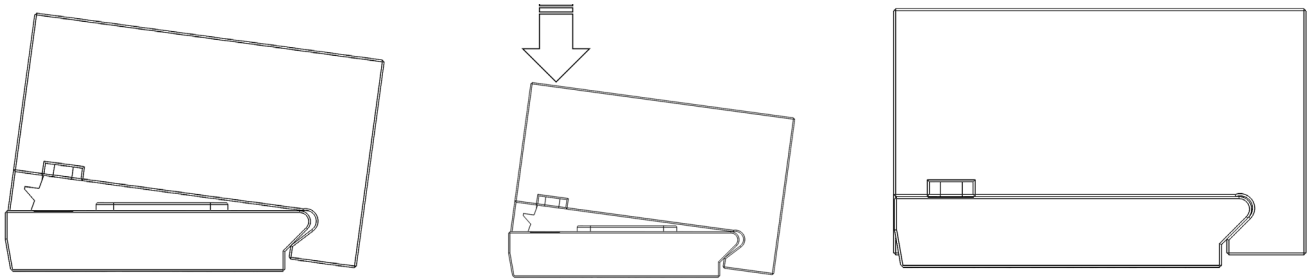
Abb. 16 Darstellung des Aufklickens der Aufsatzbacke auf die Grundbacke
