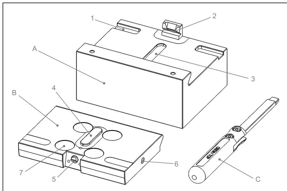
Abb. 9 Komponenten des Backenschnellwechselsystems
