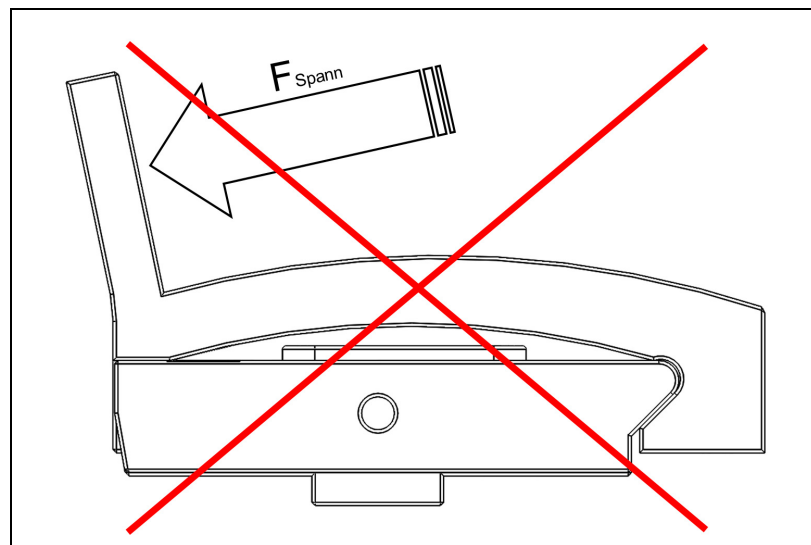
Abb. 29 Folgen einer zu geringen Bodenstärke, bzw. einer zu geringen Rückwandstärke. (Starke Deformationen der Aufsatzbacke)
